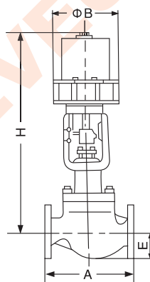
ZVA6 actuator
