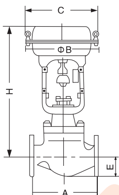
ZHA actuator
